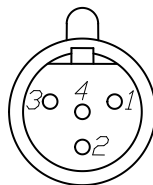
Рис.4. Нумерация контактов гнезда mini-XLR.
